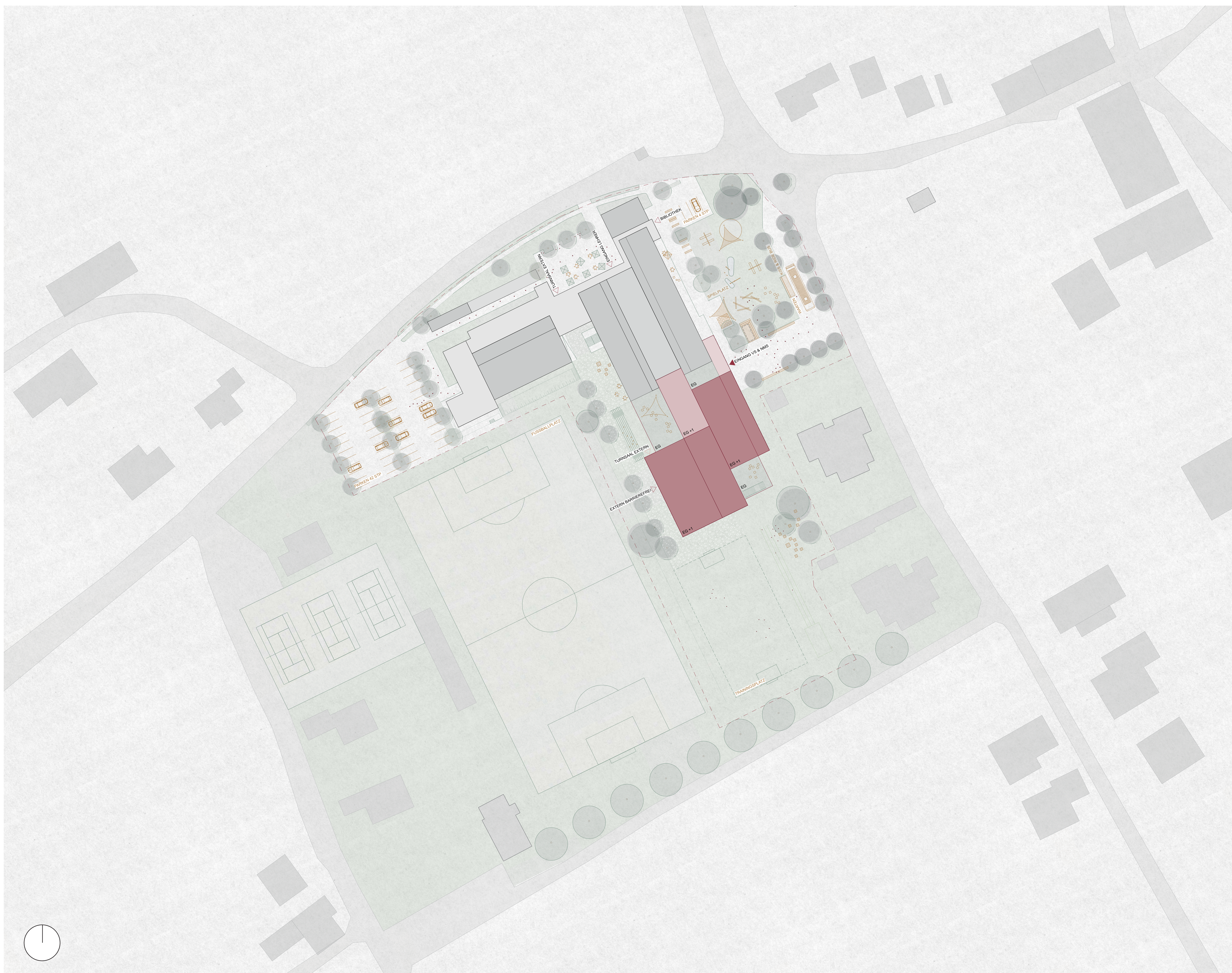
LAGEPLAN 1:500
