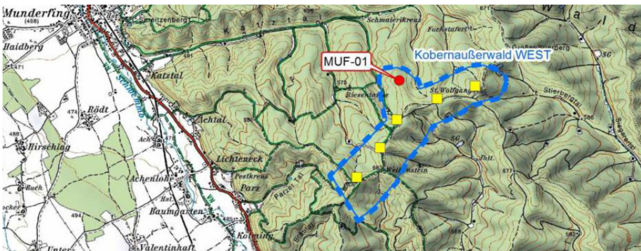
Lageplan - Standort der neuen Anlage (Foto: Energie Munderfing)
